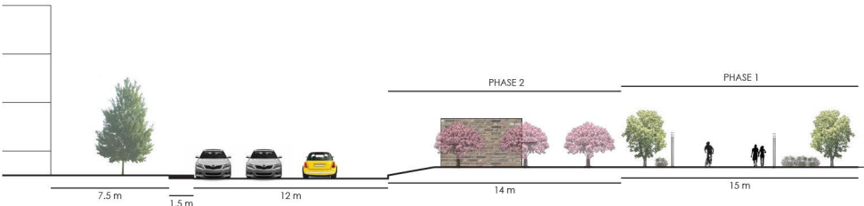
Coupe élévation, ouest du boul. du Tricentenaire
